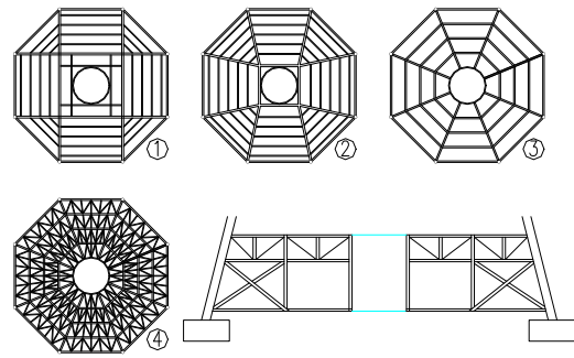
图 16 首层入口平台方案演变过程
