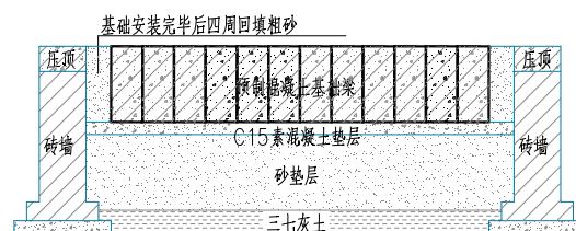
图 14 基础与夯土层间铺砂隔离构造
