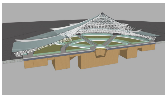
图8 洛阳明堂跨空保护方案
