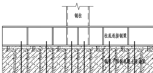
图 13 典型基础剖面图
