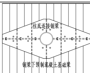
图 12 典型基础平面图
