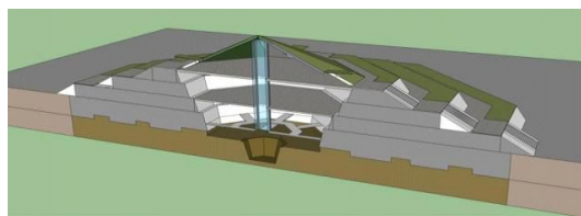
图9 洛阳明堂周边封土掩埋、中部跨空保护方案
