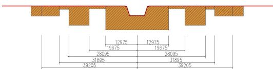
图 3 明堂遗址夯土层剖面示意图
