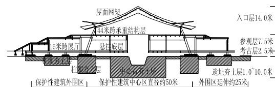
图11 洛阳明堂剖面图
