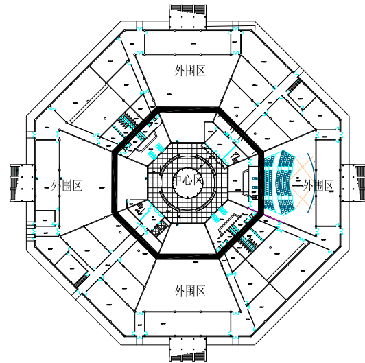
图10 洛阳明堂底层平面图
